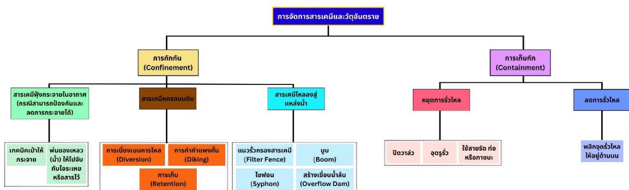
รูป 3.8 แผนภูมิการระงับการรั่วไหลหรือควบคุมการแพร่กระจายของวัตถุดิบตรายการ
